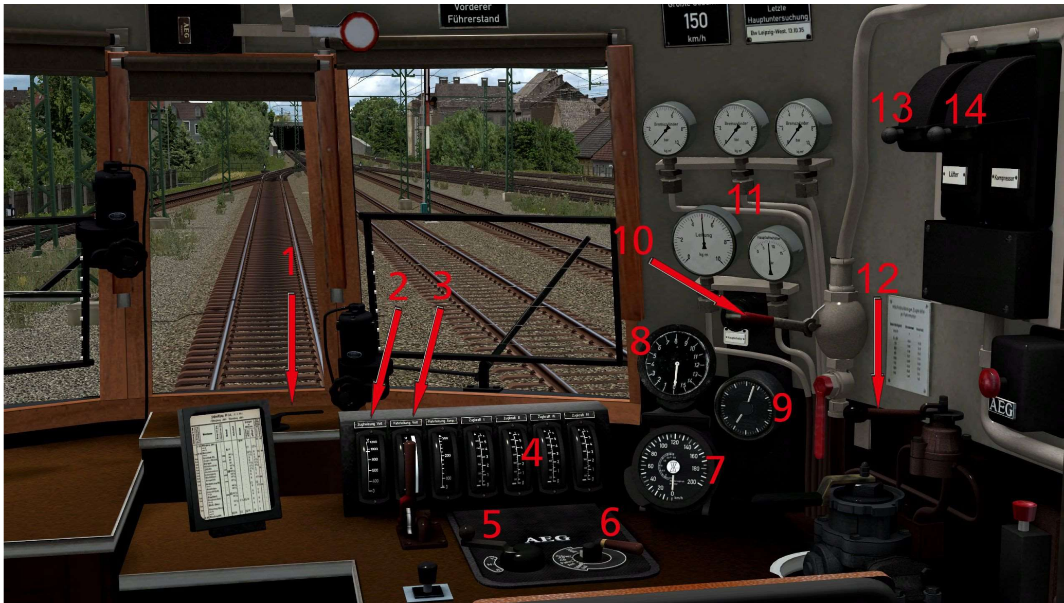
animierter und steuerbarer Führerstand – Schaubild Steuerelemente
